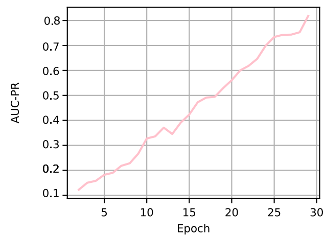
AUC-PR
