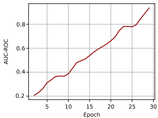
AUC-ROC
